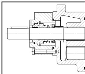
Abb. 6: Gleitringdichtung
