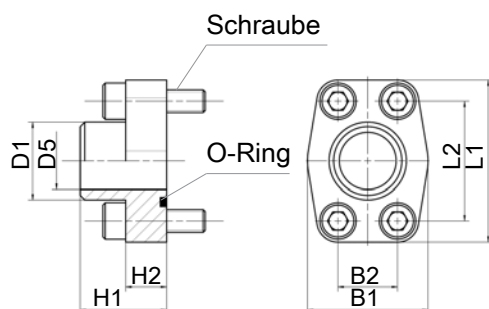
SAE-Anschweißflansch
