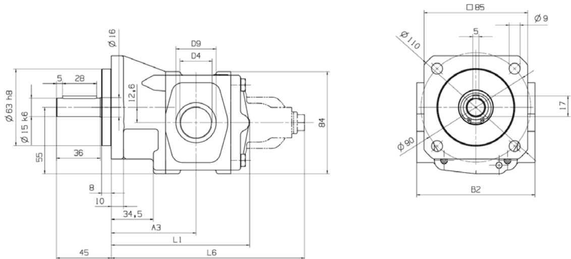
Option: Druckbegrenzungsventil
