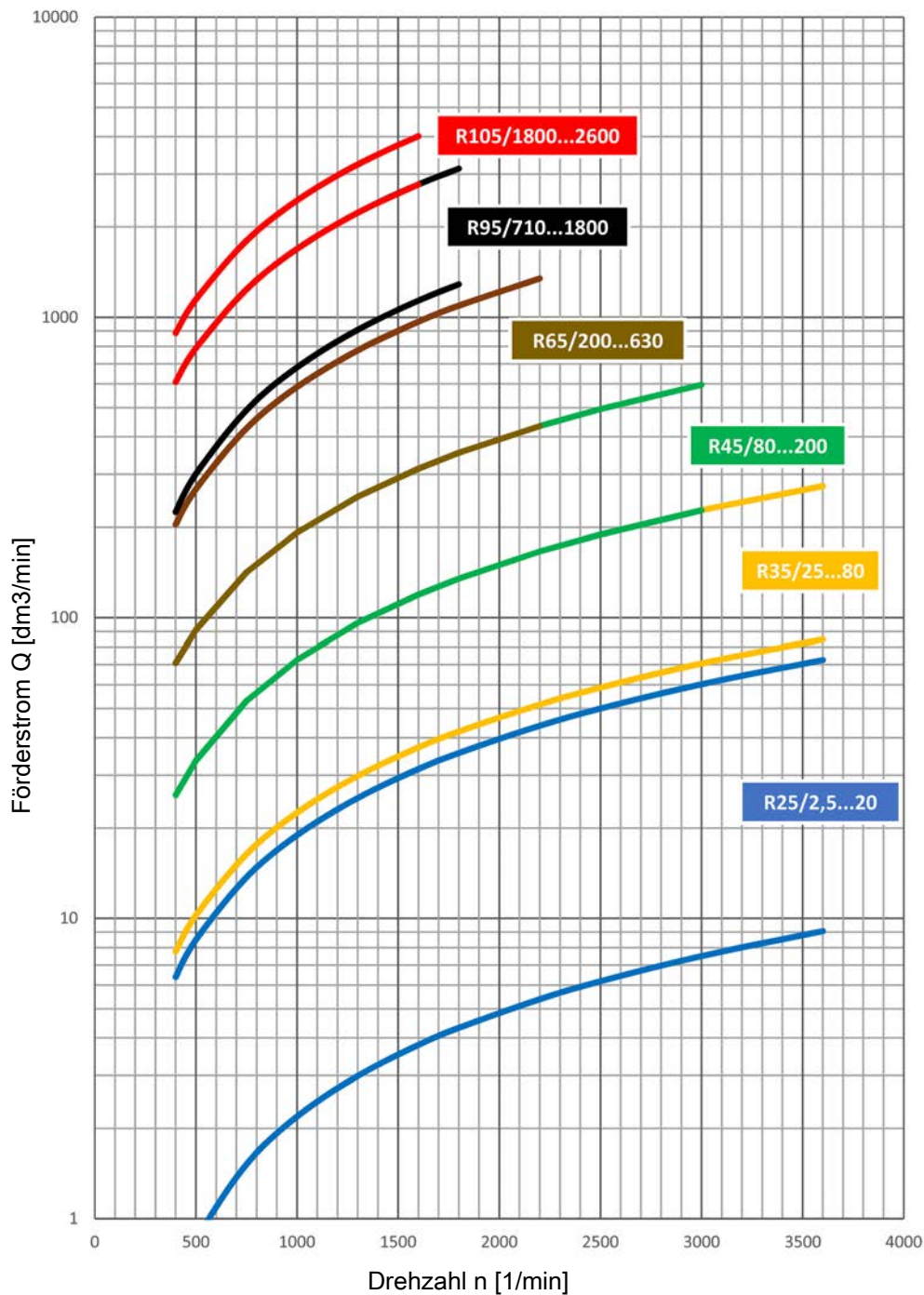
Abb. 10: Förderstrom versus Drehzahl (Werte gelten für kinematische Viskosität = 33 mm²/s und Austrittsdruck p_2 = 5 bar)
