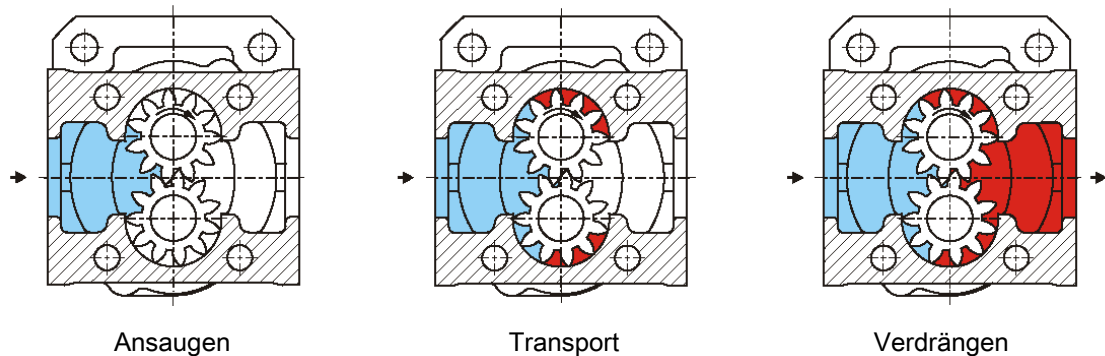
Abb. 3: Förderprinzip der Zahnradpumpe
