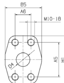
Option: SAE Anschluss
