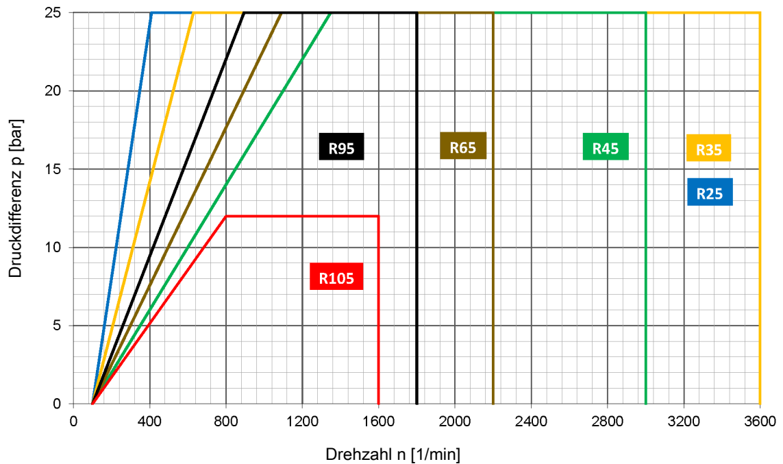
Abb. 9: Zulässige Druckdifferenz (Viskosität = 33 mm 2 /s)
